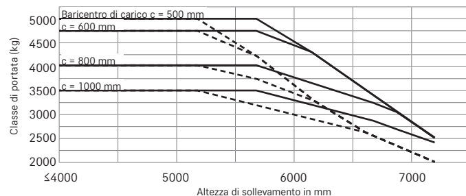
RX 60-50 montante triplex/gommatura SE semplice
