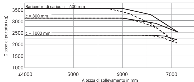
RX 60-35/600 montante triplex/gommatura SE semplice
