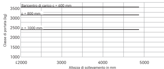
RX 60-35/600 montante telescopico/gommatura SE semplice
