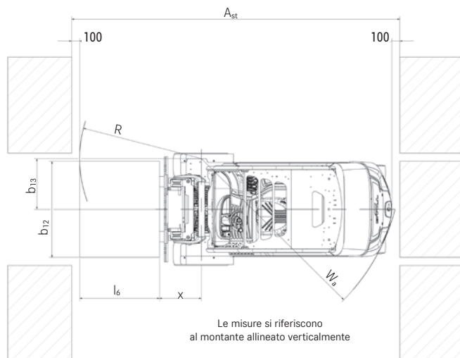
Vista dall'alto
