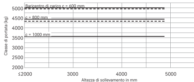
RX 60-50/600 montante telescopico/gommatura SE semplice
