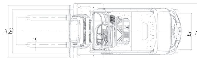
Vista dall'alto
