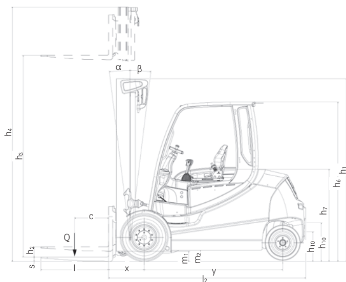
Vista laterale
