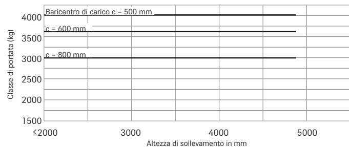
RX 60-40 montante telescopico/gommatura SE semplice
