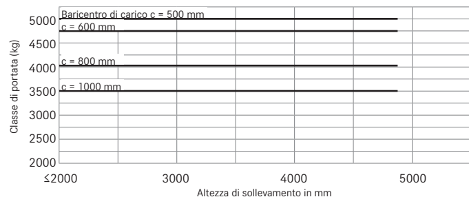
RX 60-50 montante telescopico/gommatura SE semplice
