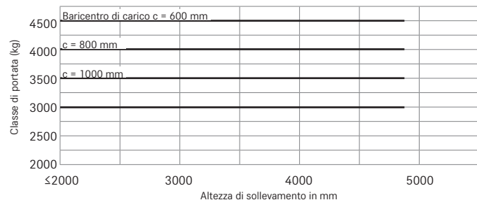
RX 60-45/600 montante telescopico/gommatura SE semplice
