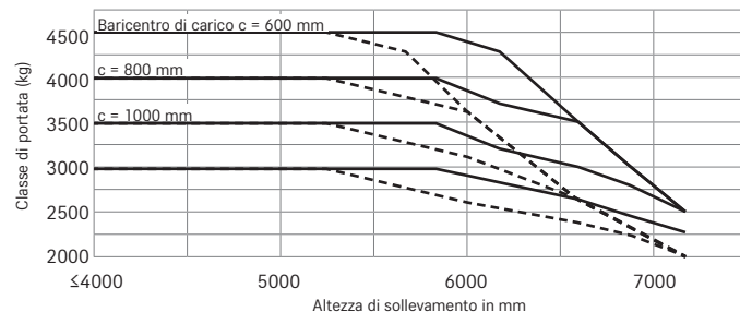
RX 60-45/600 montante triplex/gommatura SE semplice
